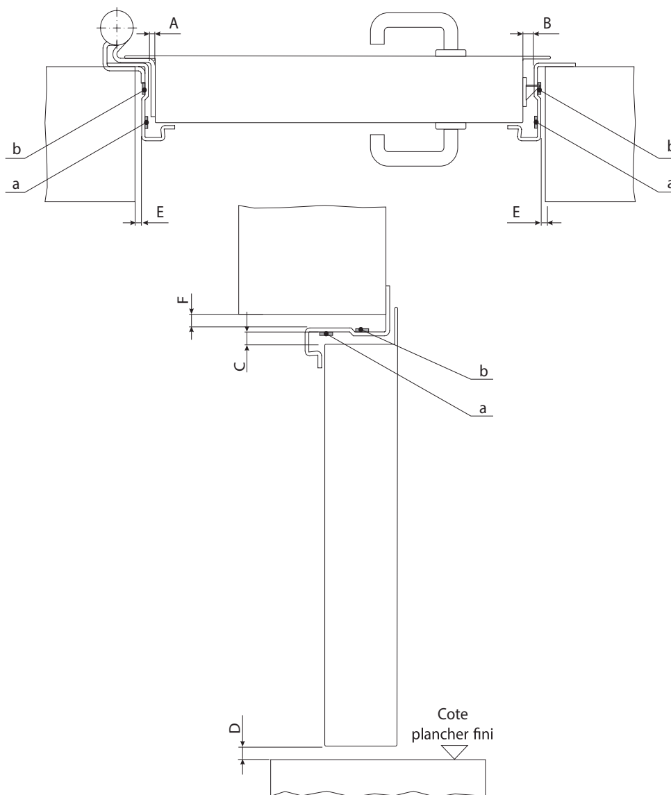
DIMENSIONS MAXIMALES
