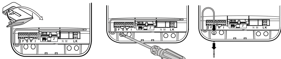
Fig. 9: Poser l'antenne
