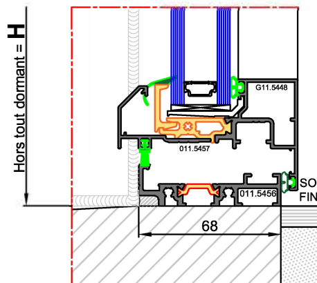
Seuil PMR
