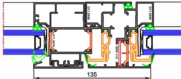
Seuil PMR
