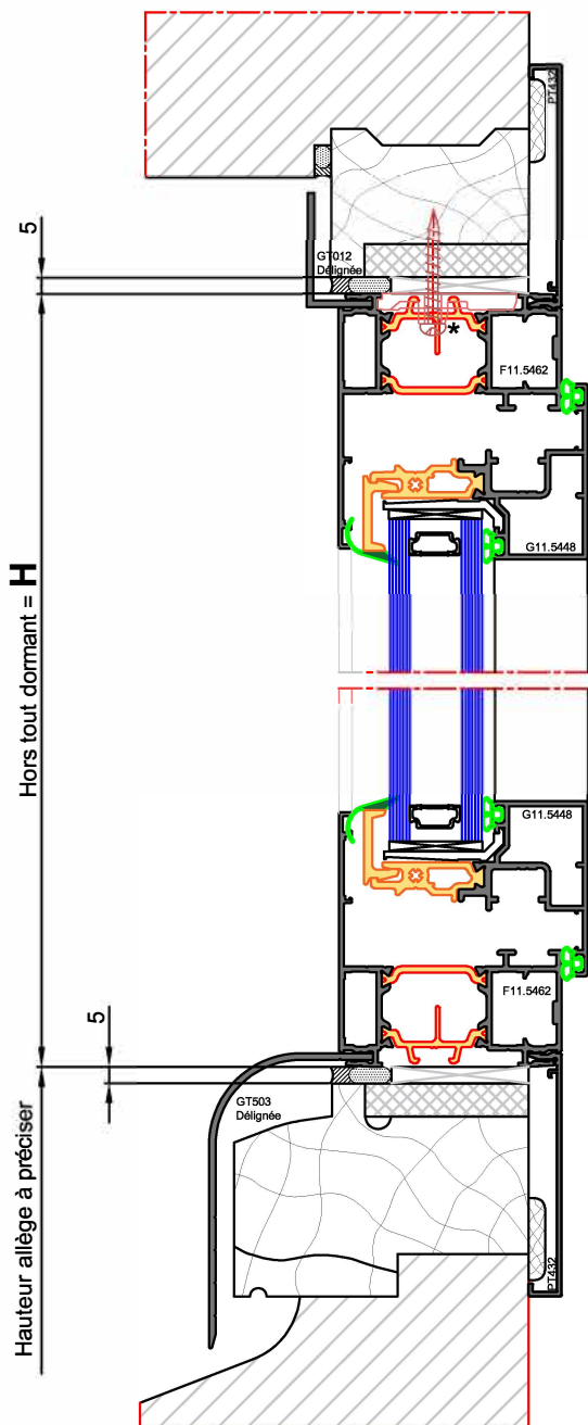
Coupe VERTICALE
