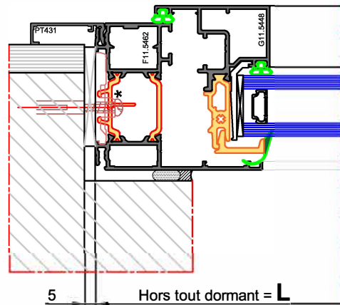
Coupe HORIZONTALE
