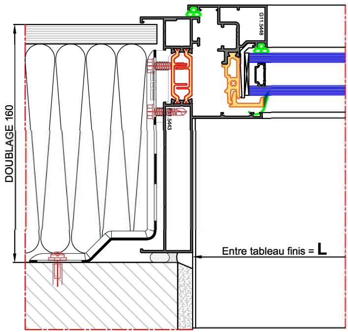
Coupe HORIZONTALE
