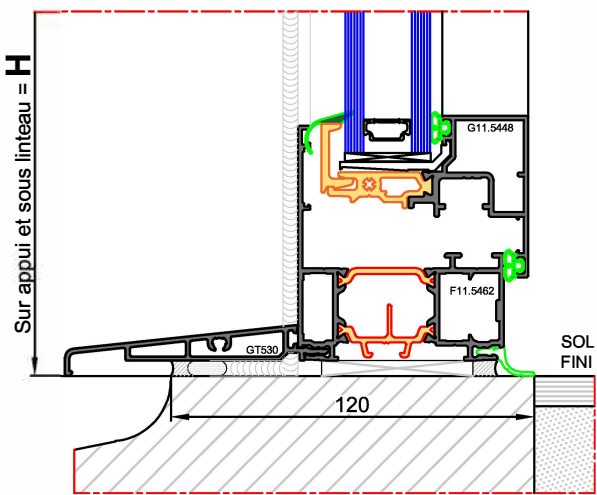
Dormant Périphérique
