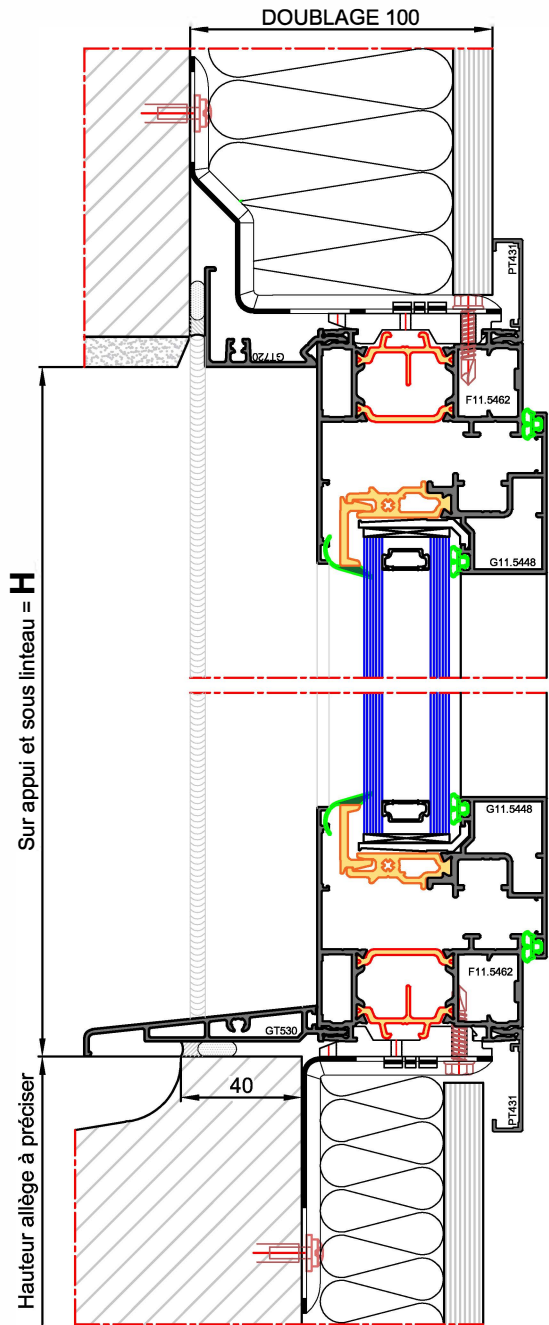
Coupe VERTICALE
