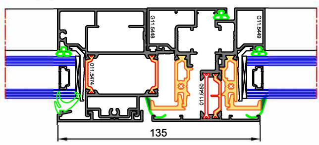
Seuil PMR
