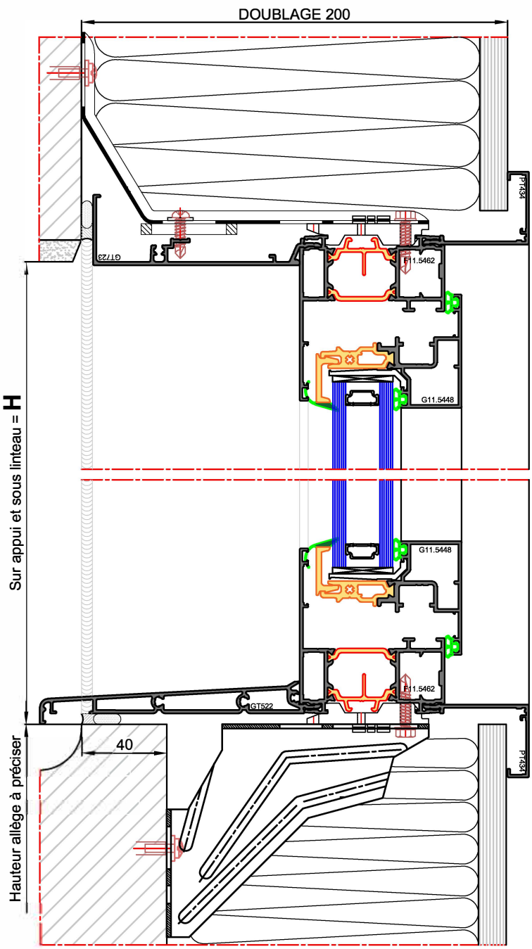
Coupe VERTICALE
