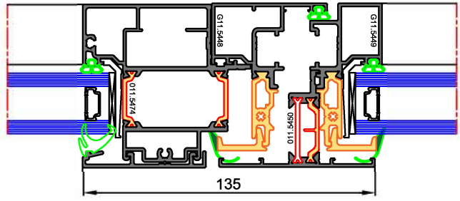
Seuil PMR
