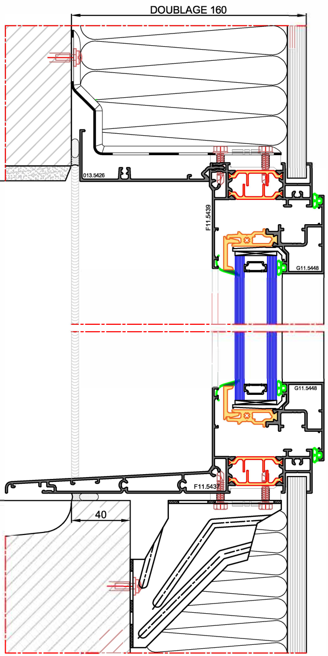
Coupe VERTICALE
