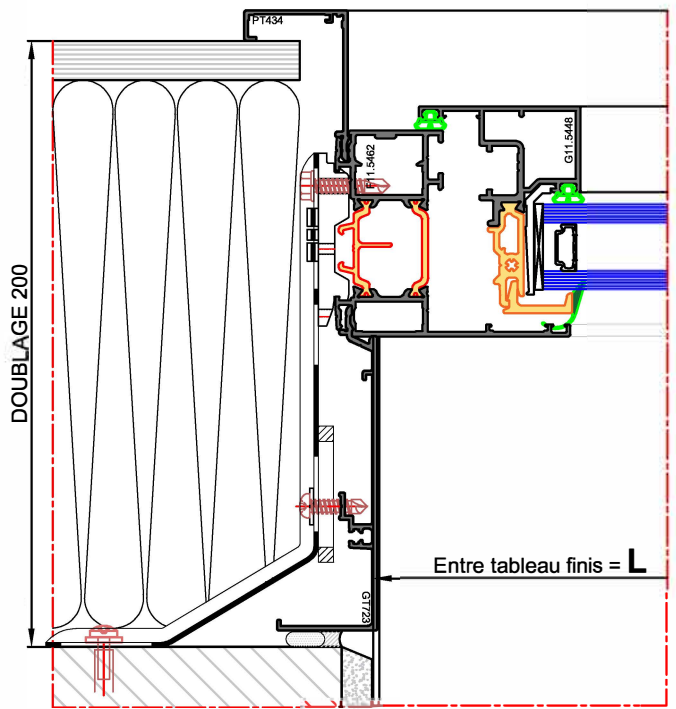
Coupe HORIZONTALE
