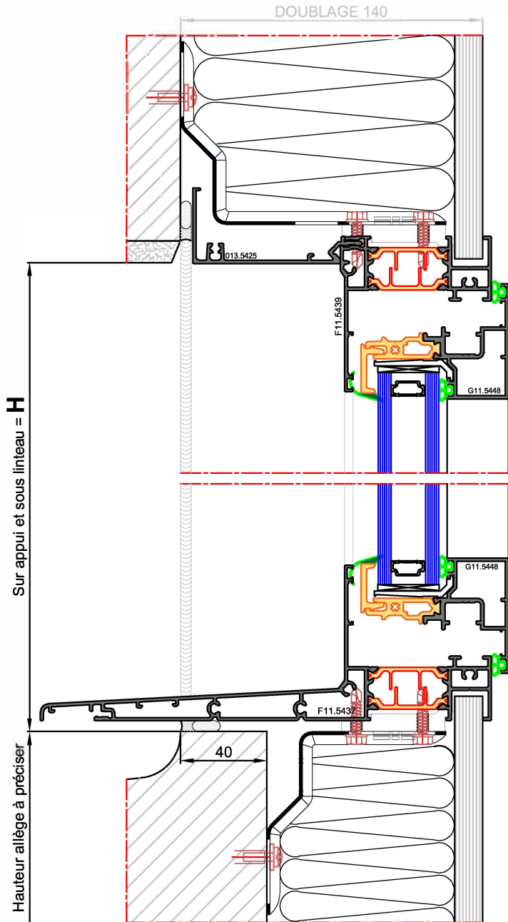
Coupe VERTICALE
