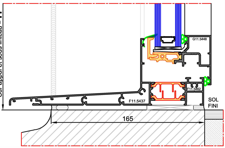
Dormant Périphérique
