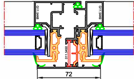
Battement CENTRAL PF serrure
