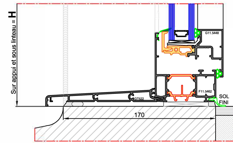
Dormant Périphérique
