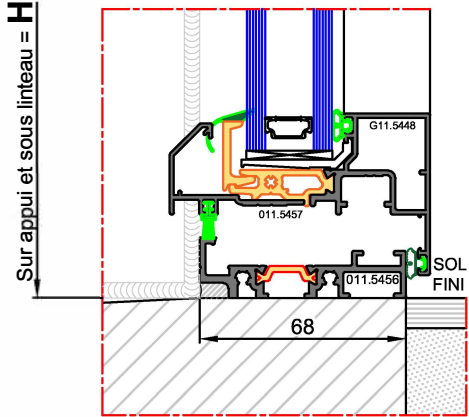
Seuil PMR
