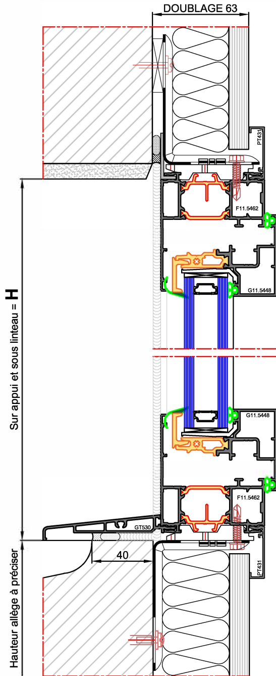
Coupe VERTICALE
