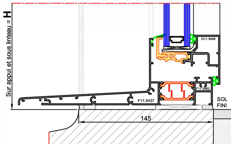
Dormant Périphérique
