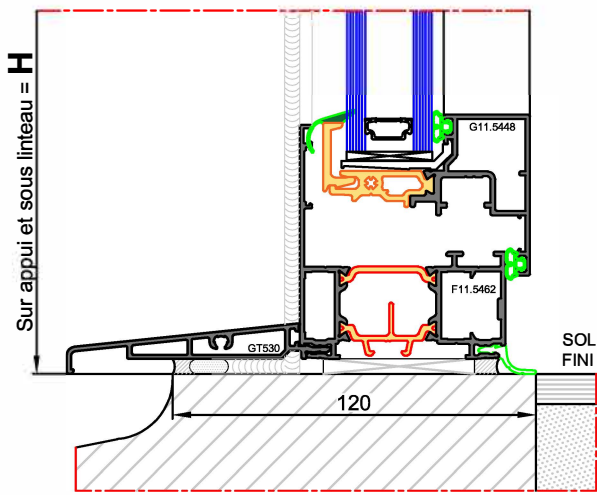
Hauteur allège à préciser
