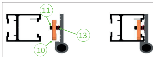
Vue de dessus: Paumelle supérieure
