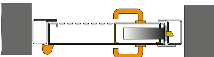
REPRESENTATION OUVERTURE EXTERIEURE
