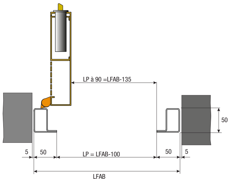
REPRESENTATION OUVERTURE INTERIEURE
