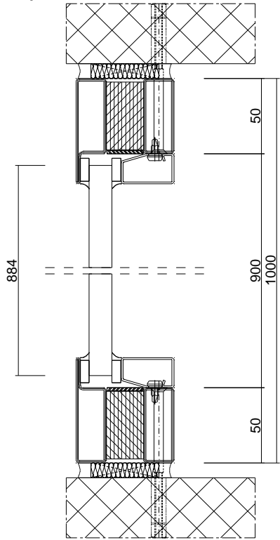
Coupe A-A M 1:3.5
