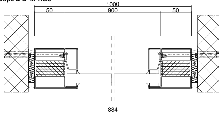
Coupe B-B M 1:3.5
