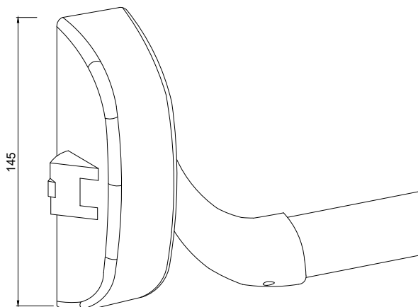
Antipanique 1 ou 3 points avec module exterieur à béquille ou à bouton
